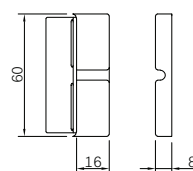
Verlengblokjes voor Verst. Sluitpl. Art. nr. 600599 (16 mm) Art. nr. 600598 (12 mm) Art. nr. 600597 (8 mm) Art. nr. 600596 (4 mm)
