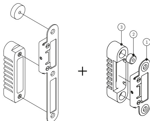
Sluitgarnituur HMB autom SKG2 Art. nr. 706105 (Din Ls/Rs) Art. nr. 706106 (Din Rs) Art. nr. 706107 (Din Ls)
