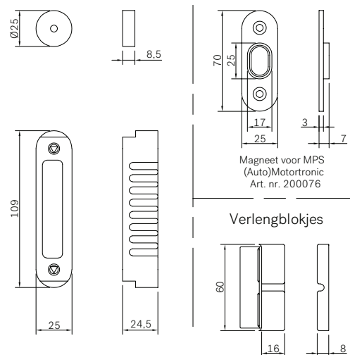
Verlengblokjes voor Verst. Sluitpl. Art. nr. 600599 (16 mm) Art. nr. 600598 (12 mm) Art. nr. 600597 (8 mm) Art. nr. 600596 (4 mm)
