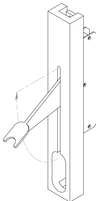
Kwartslaghendel opbouw
